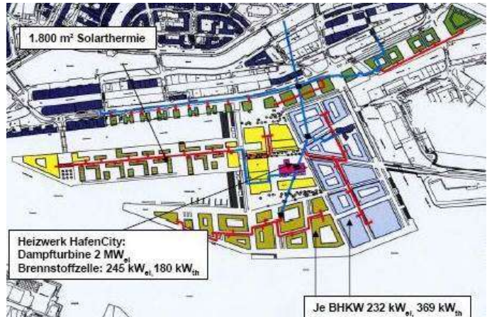
Das Energiekonzept der HafenCity
