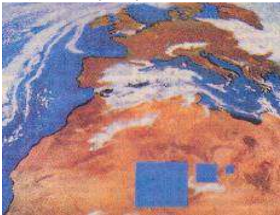
Notwendige Flächen für Solaranlagen, um den Energiebedarf Deutschlands, Europas u. der Welt zu decken
